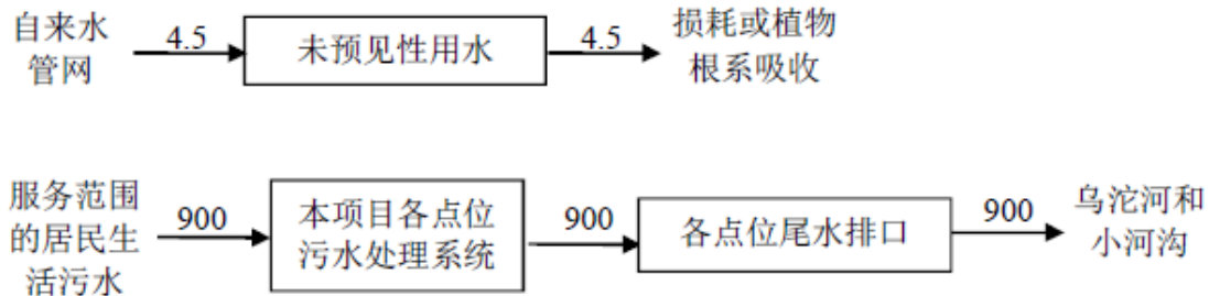
图 2-2 项目水平衡图
