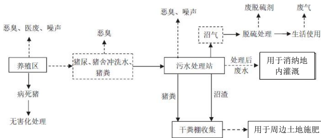
图 2.6-3 营运期工艺流程及产污位置示意图
