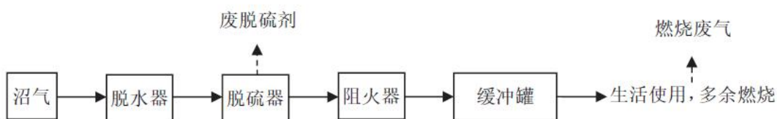
图 2.6-9 沼气净化工艺流程图
