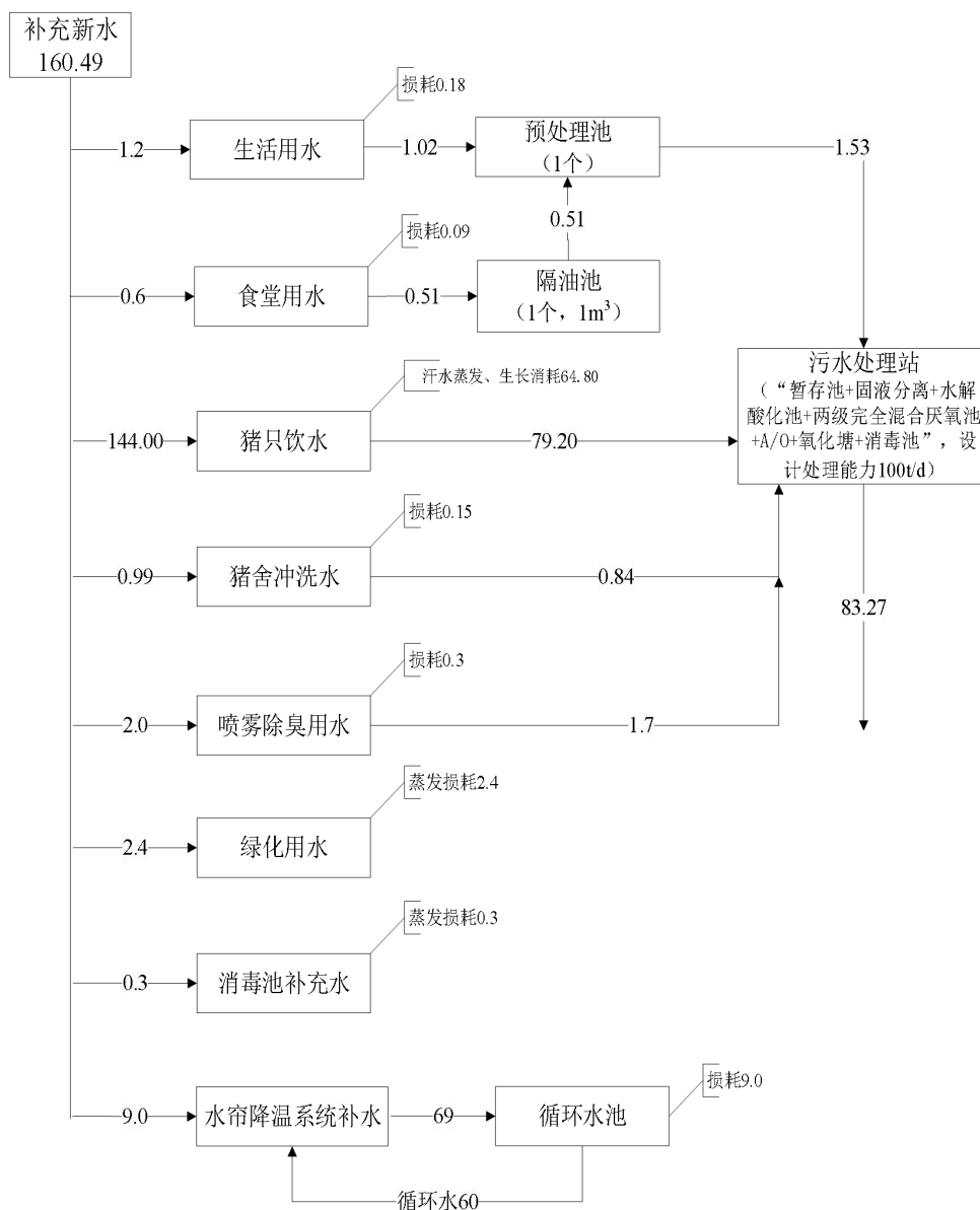
图 2.4-1 夏季全场水平衡图 (单位: m³/d)
