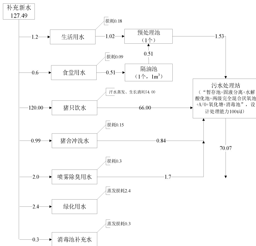
图 2.4-2 春、秋、冬季全场水平衡图 (单位: m 3 /d)
