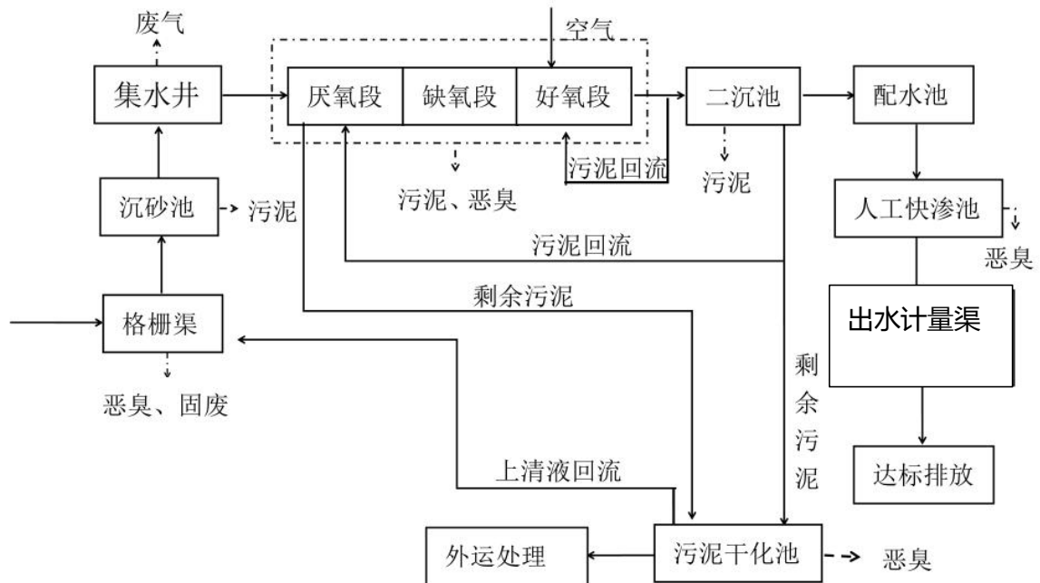
图 2-2 项目生产工艺及产污环节图
