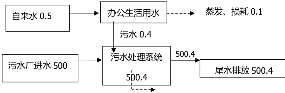
图 2-1 营运期水平衡图 单位：m 3 /d
