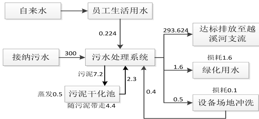
图2-1 本项目水平衡图 单位m 3 /d
