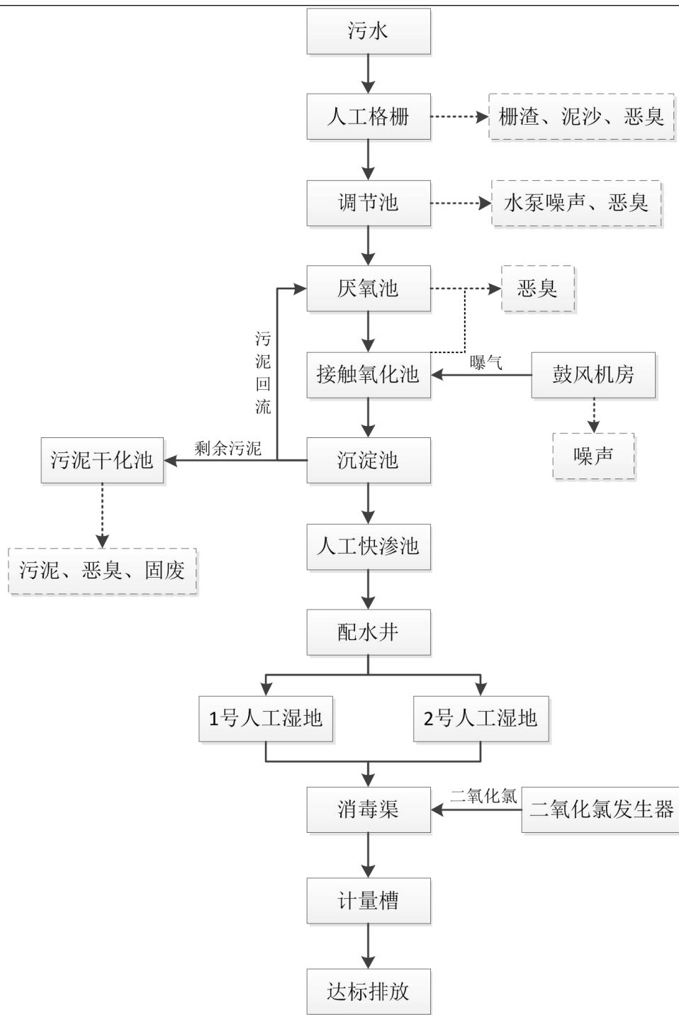
图 2-2 项目生产工艺及产污环节图
